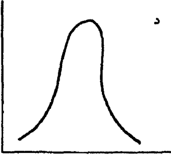
مدبب
