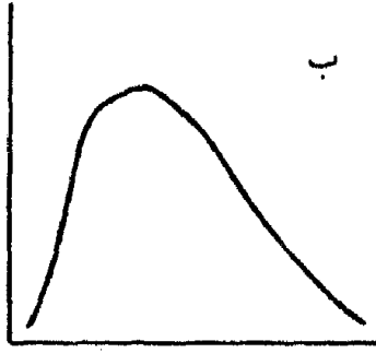
التواء موجب
