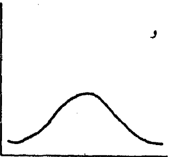
تفرطح معتدل
